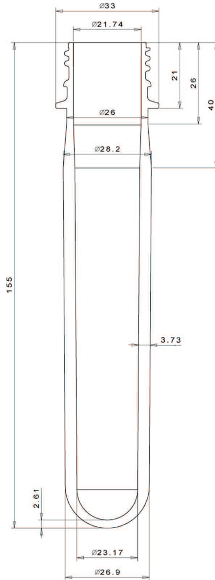
A-A View/Görünüm
